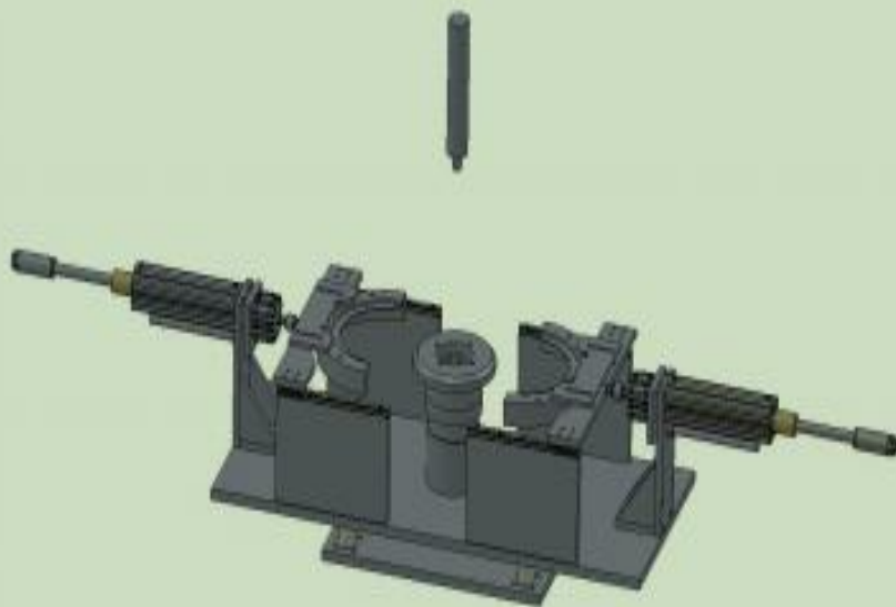
整套点焊夹具
